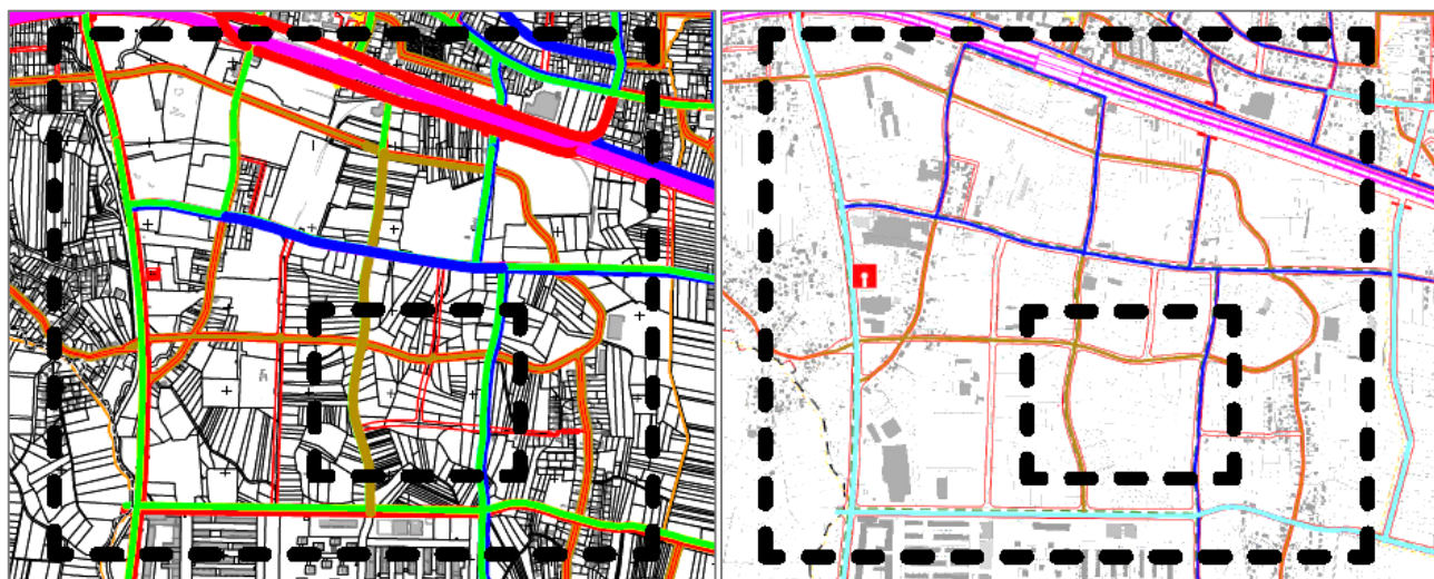
Slika 59. Usklađenje trasa prometnica sukladno UPU Gospodarska zona Sesvete – sjever osim u dijelu koji se prema ovim izmjenama i dopunama Plana nalazi unutar obuhvata UPU Jelkovec sjever
