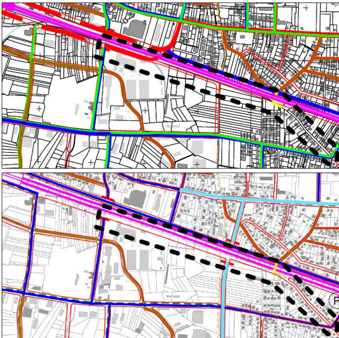
Slika 37. Prijedlog povezivanja Selnika ulice novom prometnicom do prostora Sljemena (5.2.3.)
