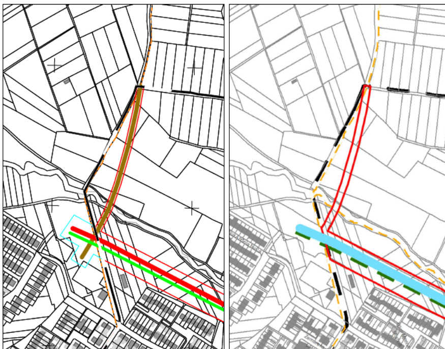
Slika 62. Izmjena kategorije koridora koji povezuje Ulicu Branovečina s planiranim koridorom Ul. R. Kolaka
